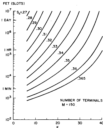
Fig. 14. FET values for a finite user population ( M = 150 ).
