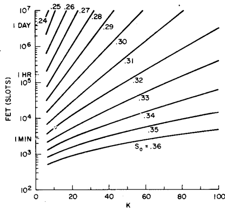
Fig. 12. FET values for the infinite population model.
