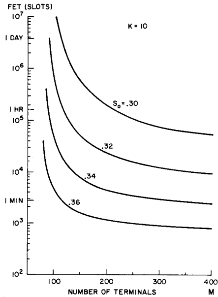
Fig. 13. FET versus M .
