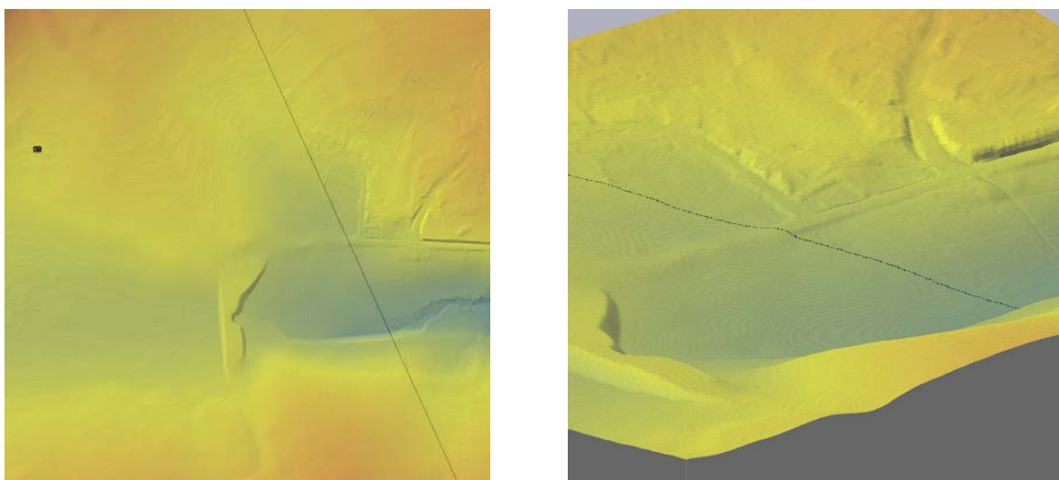
Extrait du MNT au sud-ouest de Corbigny (58) : dans la partie ouest, le MNT est issu de corrélation tandis que dans la partie est, le MNT est issu d'un traitement de données LiDAR.
