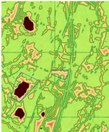
Extrait du RGE ALTI® corrélation (masque distance) le long de l'A20 au sud-ouest de la Souterraine (23). La distance d'interpolation associée à chaque nœud du MNT est ici variable en fonction de la densité des points sol mesurés par corrélation. Les zones où la distance d'interpolation est importante (zones peu denses) sont identifiées en orangé-rouge ; les zones où le MNT est issu de la BD ALTI® version 1.0 apparaissent en marron (code 253).
