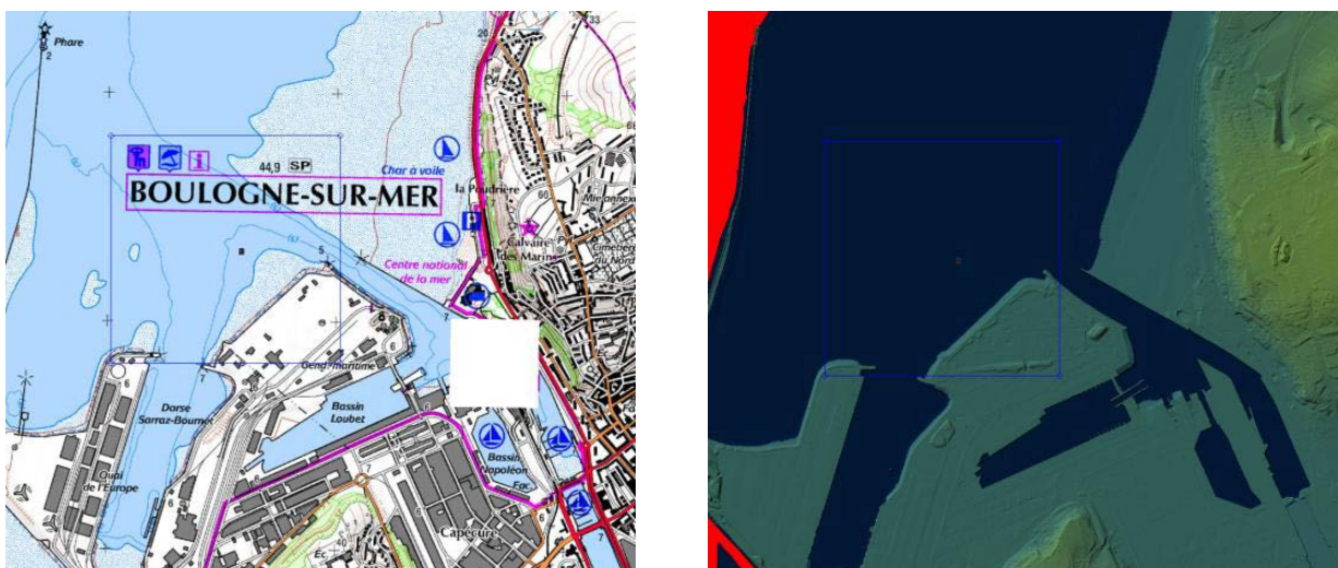
Mise à plat du port de Boulogne-sur-Mer dans le MNT issu d'acquisitions LiDAR.
