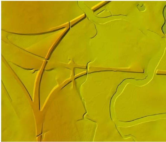
Ouvertures des ponts (franchissement des réseaux hydrographique, routier ou ferré) sur un extrait de MNT
